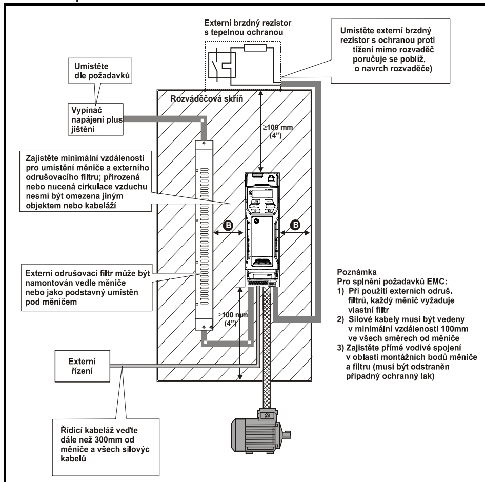
Obr. 3-12 Uspořádání rozváděče
