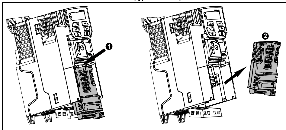
Obr. 3-7 Demontáž volitelného SI modulu (typ. vel. 2 až 4)
